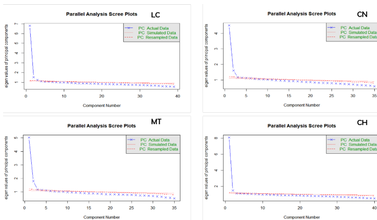
FIGURA 1 - Scree plot da análise paralela das provas do Enem 2017
