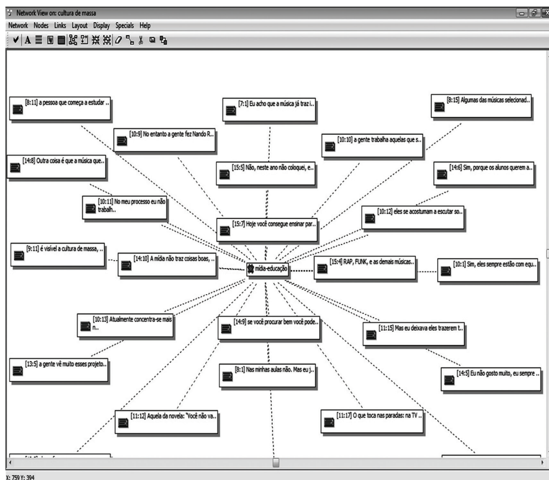
Figura 2 – Categorização
